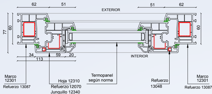
Detalle 2
