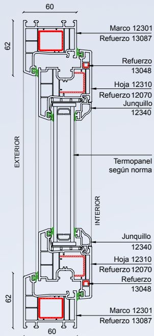
Detalle 1
