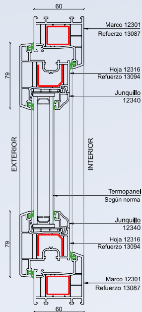
Detalle 1
