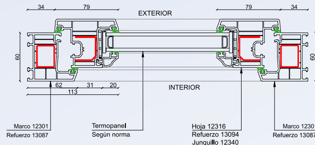
Detalle 2
