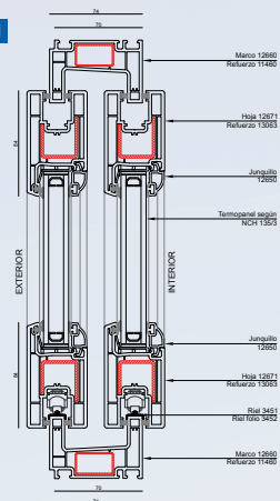
Detalle 1
