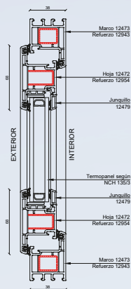
Detalle 3
