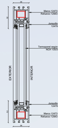
Detalle 2
