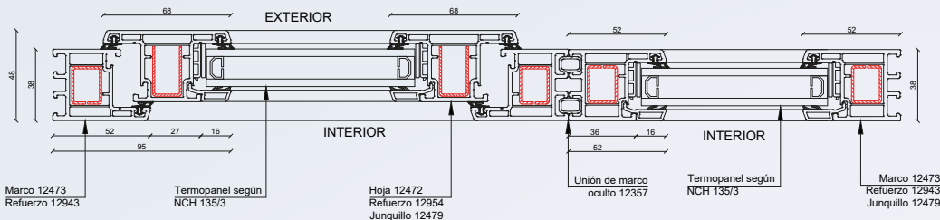
Detalle 3
