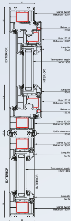
Detalle 1
