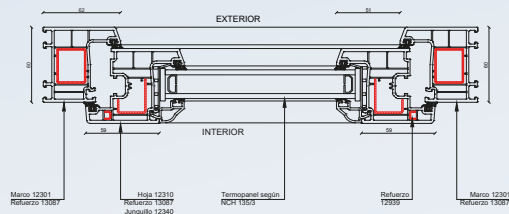
Detalle 3
