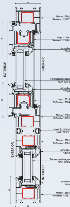
Detalle 1
